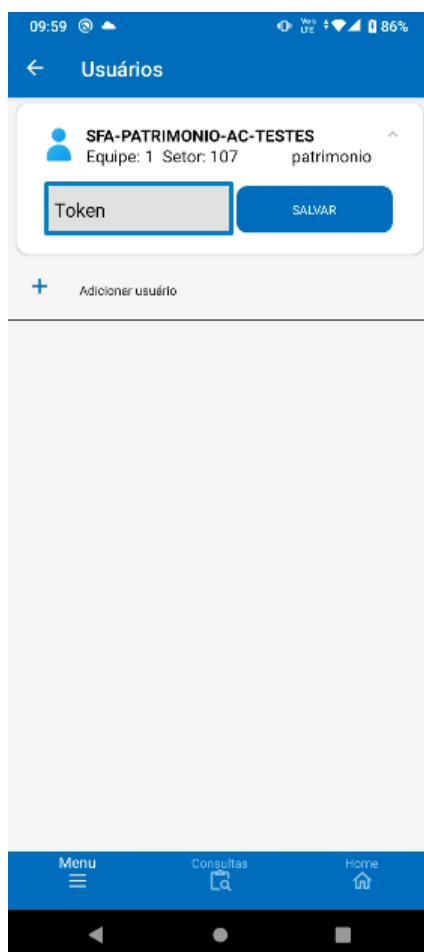
Figura 7: Token.
